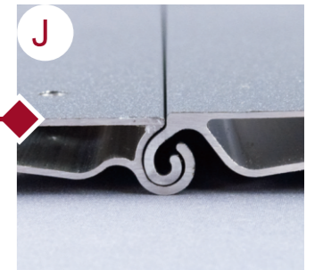
J 門片特殊串接(後柳)設計可提升平滑捲動及耐用
