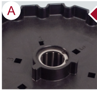
A 快速捲門捲軸轉輪中心採用不鏽鋼滾針軸承設計
