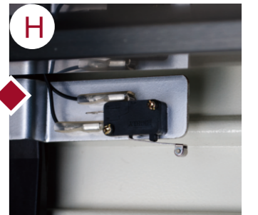
H 防過捲擋片裝置可防止捲門過捲故障
